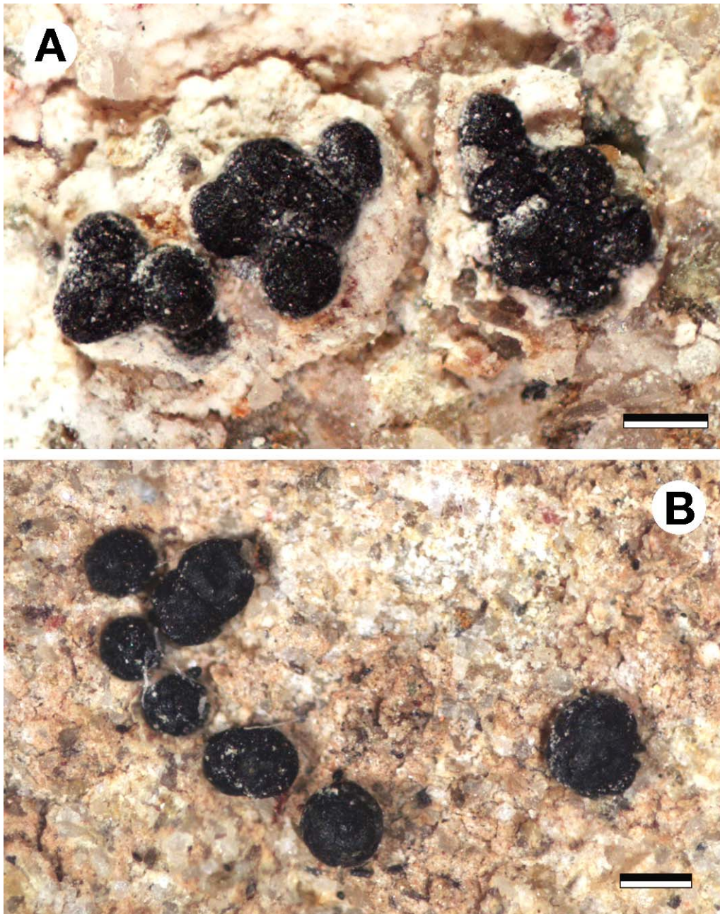
Fig. 5.- A , Sarcopyrenia cylindrospora (BCN-lich. 15651). Ascomas parcialmente hundidos en talo alterado de Aspicilia calcarea . B , Sarcopyrenia gibba var. geisleri (BCN-lich. 2042). Ascomas sobre zonas del substrato alteradas por el hongo, en las que ha desaparecido totalmente el talo del hospedande (probablemente Caloplaca aurantia ). Escala: A y B = 300 \mu m.
