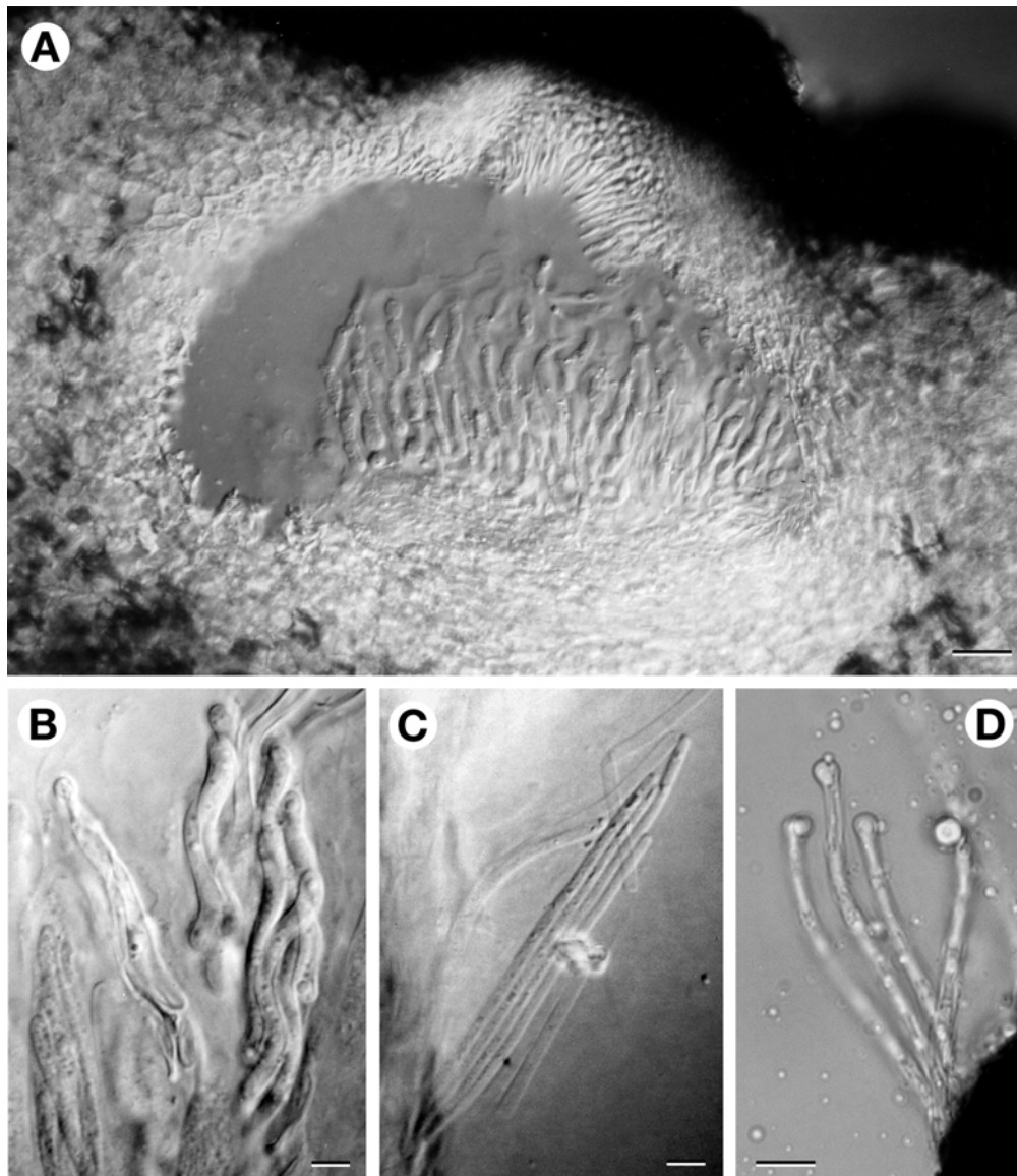
Fig. 1.- A, sección de ascoma inmaduro de Sarcopyrenia gibba var. geisleri , donde se aprecian los filamentos interascales formados previamente a la maduración de los ascos (BCN-lich. 2042). B, ascósporas de Sarcopyrenia gibba var. gibba (Holótipo). C, ascóspora de Sarcopyrenia beckhausiana (BCN-lich. 4146). D, vista de un extremo de las ascóspora de Sarcopyrenia baetica (Holótipo). Escalas: A = 20 \mu m; B, C y D = 5 \mu m.
